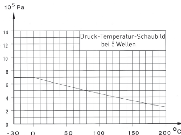
DN 015-500
