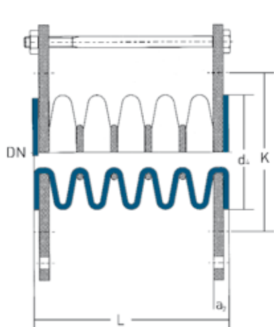
DN 015-500
